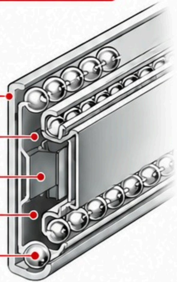
Diagrama da estrutura da corrediça
