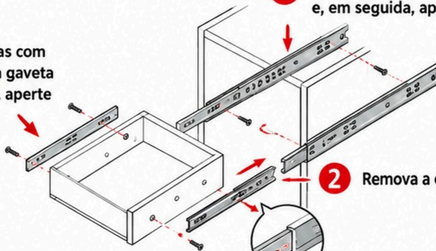
Diagrama da posição da corrediça
